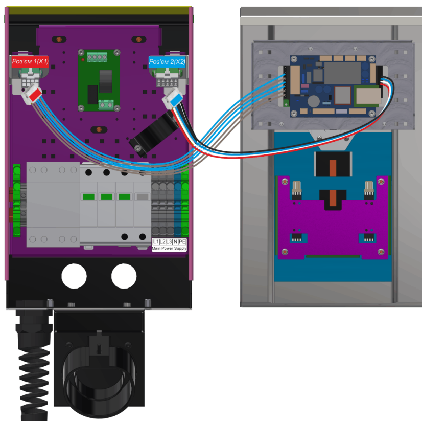
Рис.11 - Від'єднання роз'ємів мініфіт
