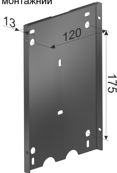
Кронштейн монтажний
