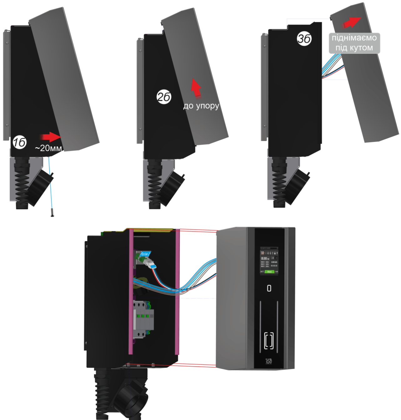
Рис. 10 – Зняття лицевої обшивки зарядної станції
