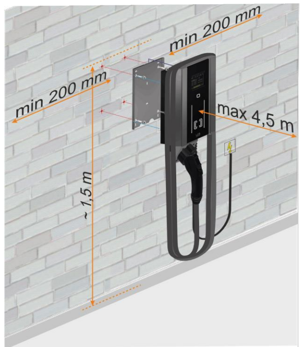
Рис.4 - Рекомендації щодо габаритів монтажу на стіну
