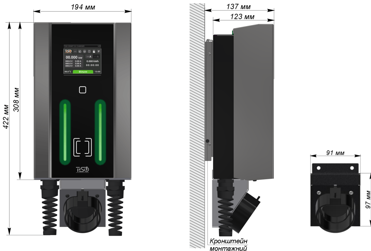
Рис.3 - Габарити та загальний розмір зарядного пристрою для електроавтомобіля
