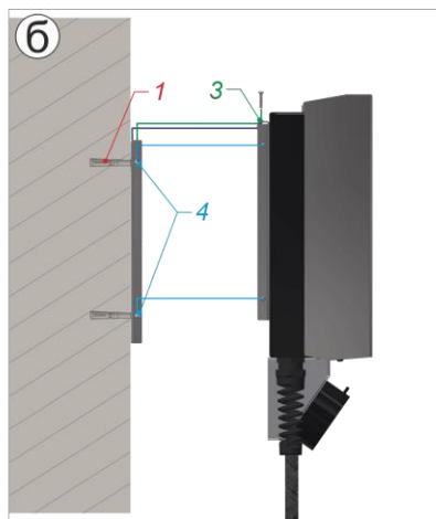
Рис.7 – Монтаж зарядної станції на стіну
