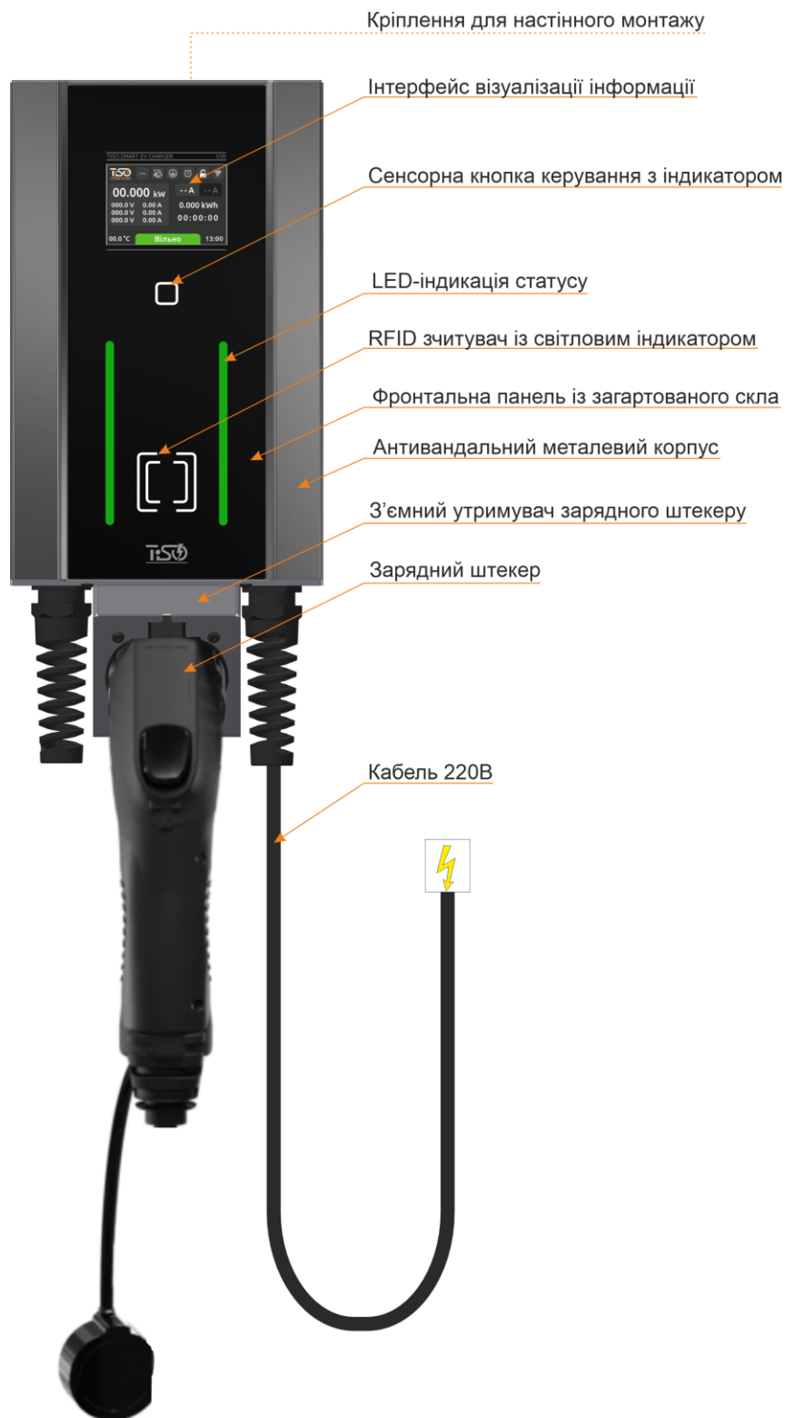
Рис.2 – Загальний вигляд станції
