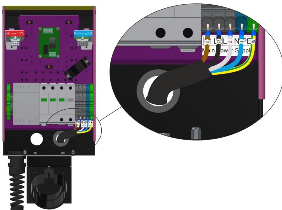
Рис.12 – Підключення кабелю живлення
